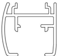
F. E-WJ - Wall jamb
