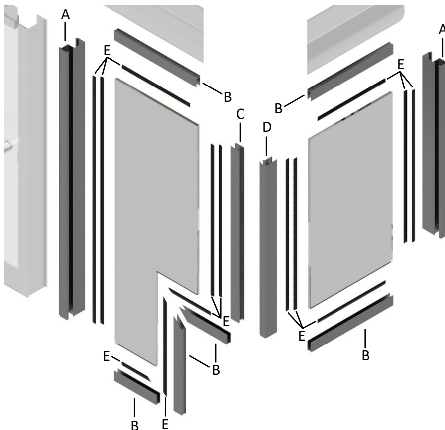
A. E-ILPJ – Slider inline post jamb
