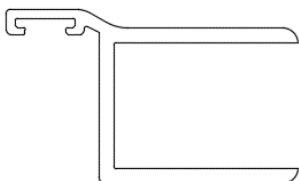
F. E-SJSFL - Semi-frameless strike jamb
