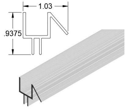
1/2" Glass Door Sweep 98" M-P-12DS
