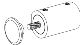
M. C-GTW – 2" square GTW clamp
