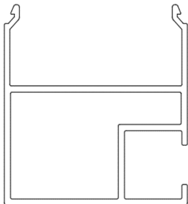
B. E-ILPJ – Slider inline post jamb
